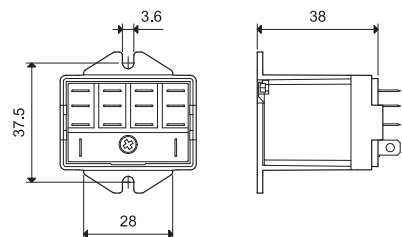
056.45 mit Relais
