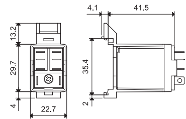
056.27 mit Relais
