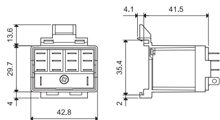
056.47 mit Relais
